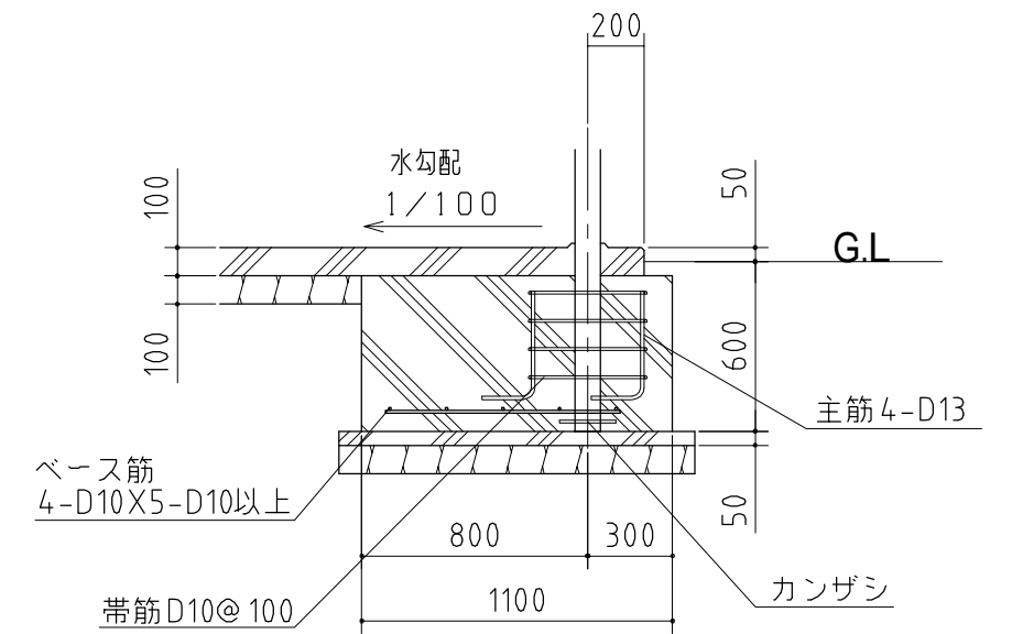
A-A' 断面
